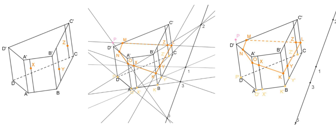
Obrázek 1 - 3: Řez tělesa (v Geogebra)
