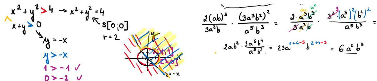
Obrázek 4 - 5: Ukázky Whiteboard
